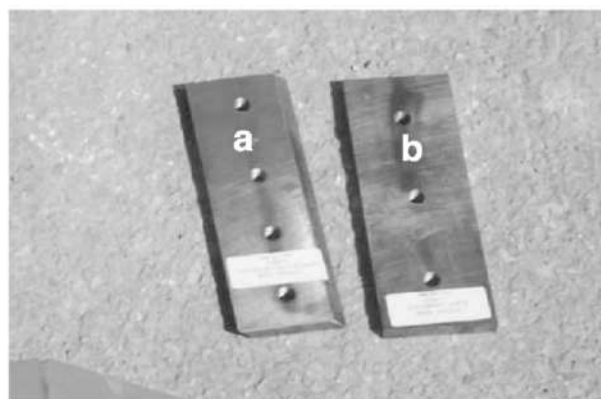
Роторный нож (a) Стационарный нож (b)
