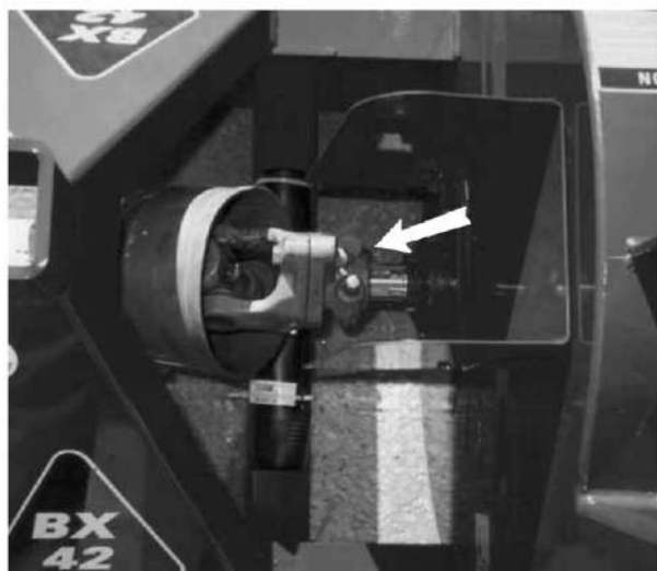
Рис. 30. Расположение срезного штифта.
