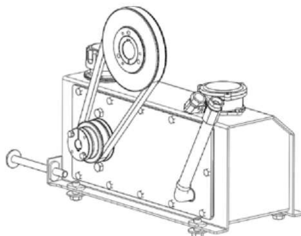
Рис. 39. Гидравлический приводной блок для модели VX62R.
