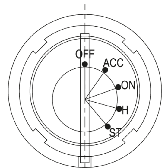
Рис. 9.1. Замок зажигания.
