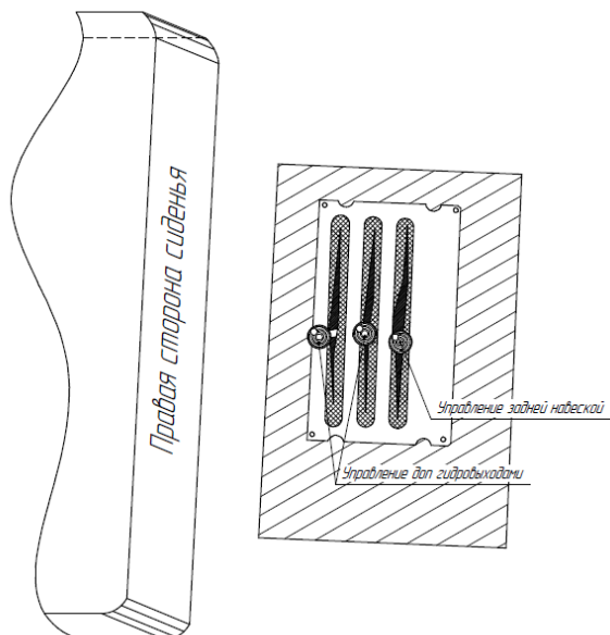
Рис. 9.6. Рычаги гидравлического подъемника и управления доп. гидровыходами.
