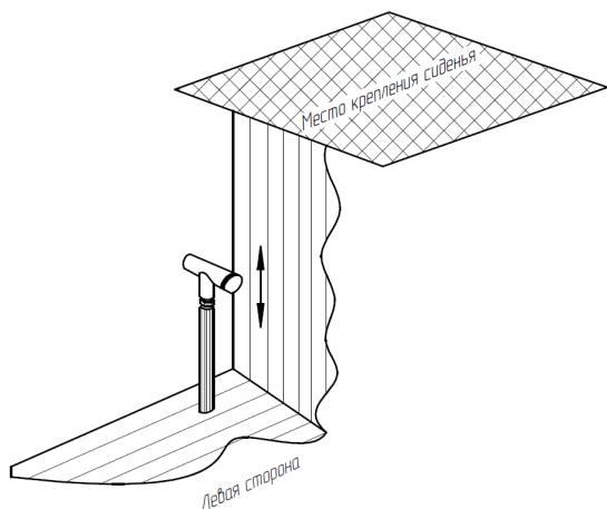
Рис. 9.8. Рычаг включения переднего моста.
