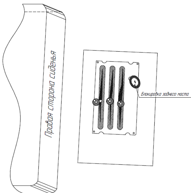
Рис. 9.7. Рычаг блокировки заднего моста (дифференциала).
