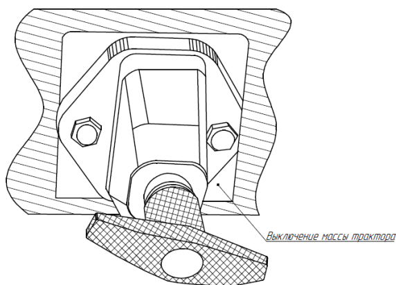
Рис. 9.9. Ручка выключения массы трактора.
